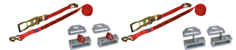
Ladungssicherung mit Gabelklemmen und Spanngurten
