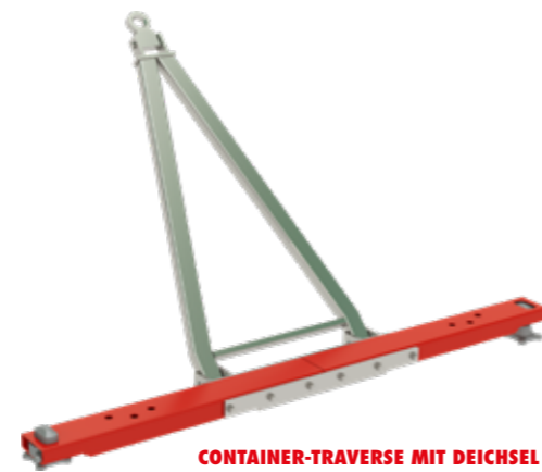
CONTAINER-TRAVERSE MIT DEICHSEL BESTELL-NR.: 92 000 226-T2
