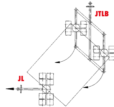
Beispiel: Kurvenfahrt bei beengten Platzverhältnissen Lenkschlag bis 45° möglich
