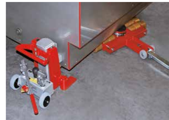
JH 15 G plus im Einsatz in Kombination mit dem JL 9 K
