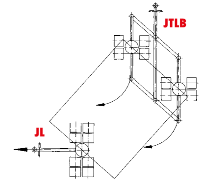
Beispiel: Kurvenfahrt bei beengten Platzverhältnissen Lenkschlag bis 45° möglich
