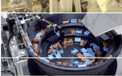
Zuführen von Klemmleisten
