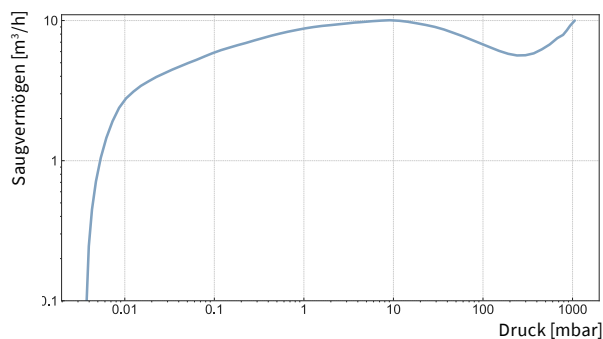
Saugvermögenskurve
