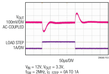
Bild 3: Mit minimalen Ausgangskondensatoren ( 2 \times 4,7 \mu\text{F} Keramik) bringt es der LTM8074 auf ein schnelles Lastsprungverhalten (bei 12 V Eingangs- und 3,3 V Ausgangsspannung).
